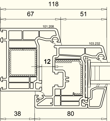
OptiLine VEKA 70 AD
